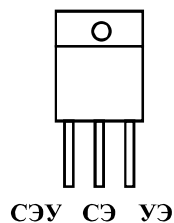
Расположение выводов симисторов ВТ139-600, ВТВ16-6, ВТА41-600
