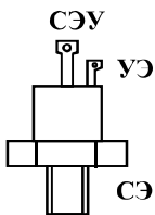
Расположение выводов симисторов ТС16, ТС122, ТС132, ТС142, ТС171
