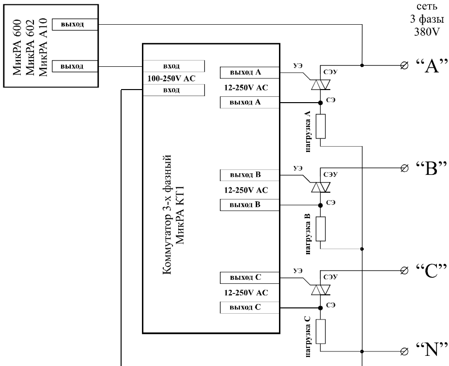
Схема подключения 3-х фазной нагрузки к регуляторам температуры МикРА с использованием коммутатора МикРА КТ1 и симисторов ТС16, ТС122, ТС132, ТС142, ТС171, ВТ139-600, ВТВ16-6, ВТА41-600
