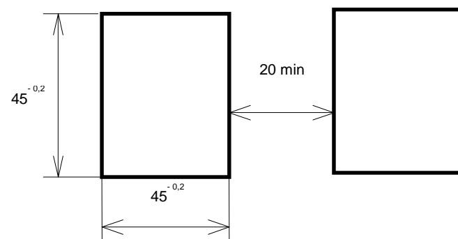
Рис.1. Вырез в щите для крепления прибора.
